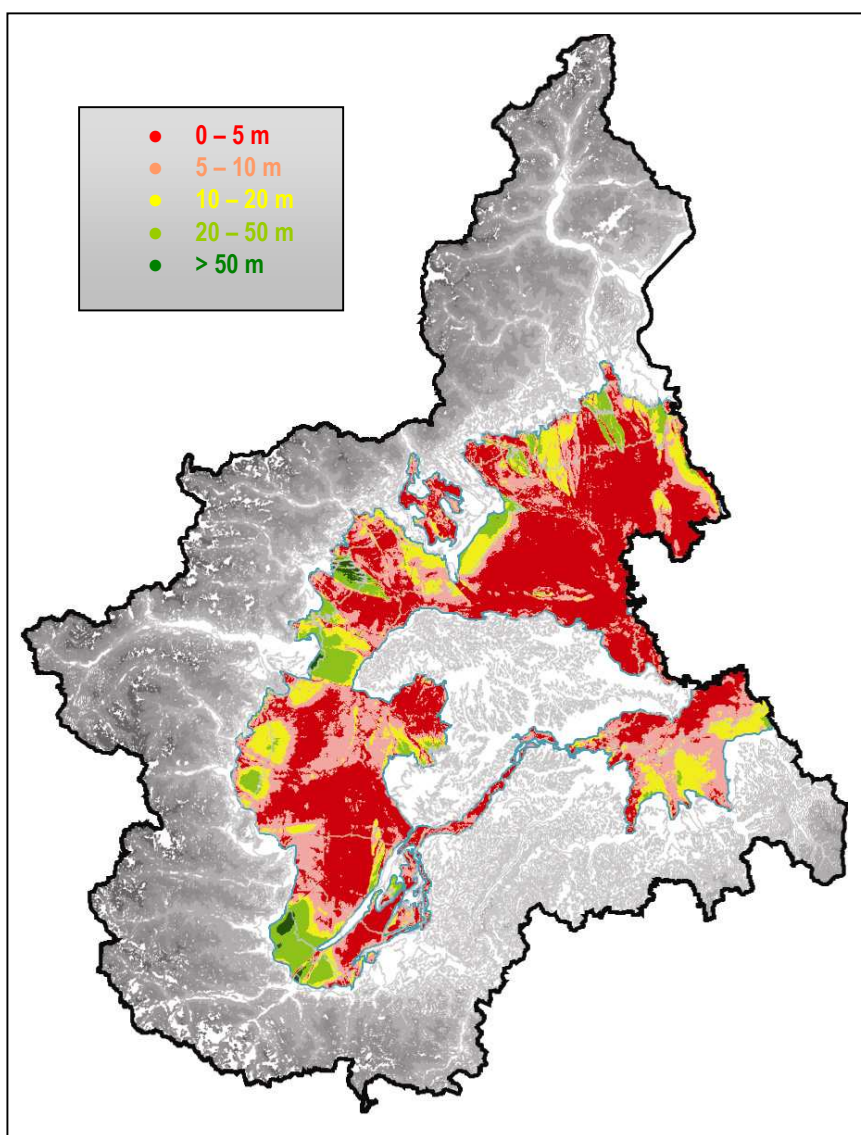
Carta della soggiacenza della falda superficiale (cf. CD-ROM - allegato II.2) Depth to groundwater map (see CD-ROM - allegato II.2)
