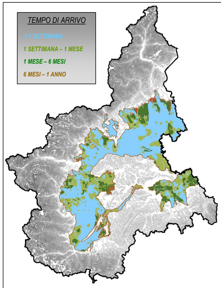
Carta del tempo di arrivo di un inquinante idrotrasportato (T.O.T.) (cfr. CD-ROM - allegato IV.2) Time of arrival of a water-carried pollutant (Time of Travel method) (see CD-ROM - allegato IV.2)
