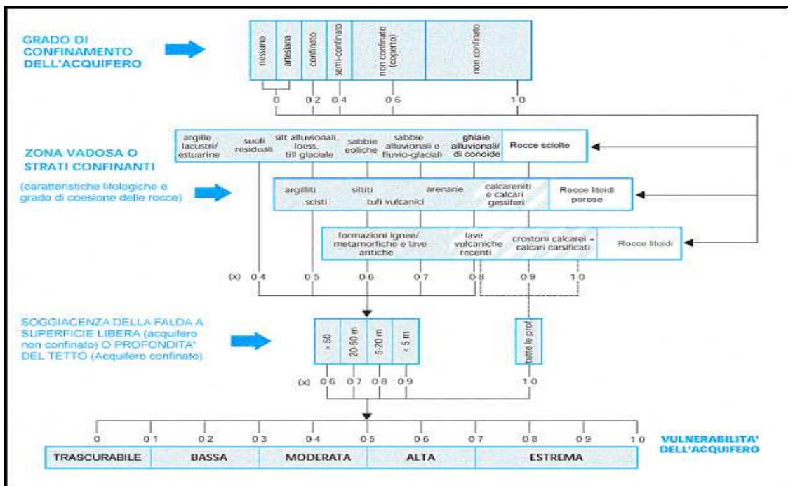
Metodo empirico G.O.D. per una valutazione rapida della vulnerabilità dell'acquifero all'inquinamento (Foster e Hirata, 2002) Empiric G.O.D method for a fast aquifer vulnerability assessment (Foster & Hirata, 2002)
